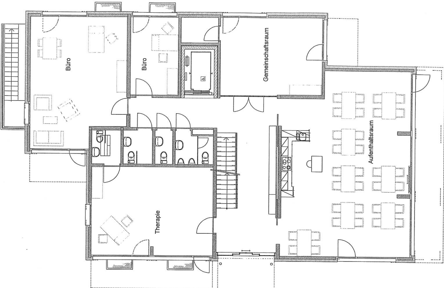
Erdgeschoss Übersichtsplan
